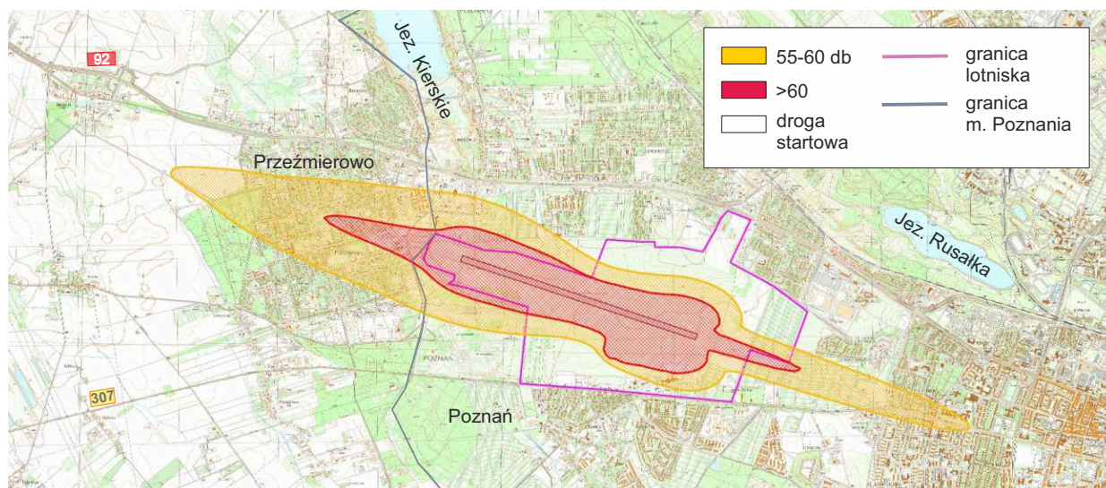
Mapa 5.2. Izolinie długookresowego średniego poziomu dźwięku A wyznaczonego w ciągu wszystkich dob w roku 2013 ( L_{DWN} ) emitowanego przez samoloty podczas wykonywania operacji lotniczych /wg AKUSTIX Sp. z o.o./
