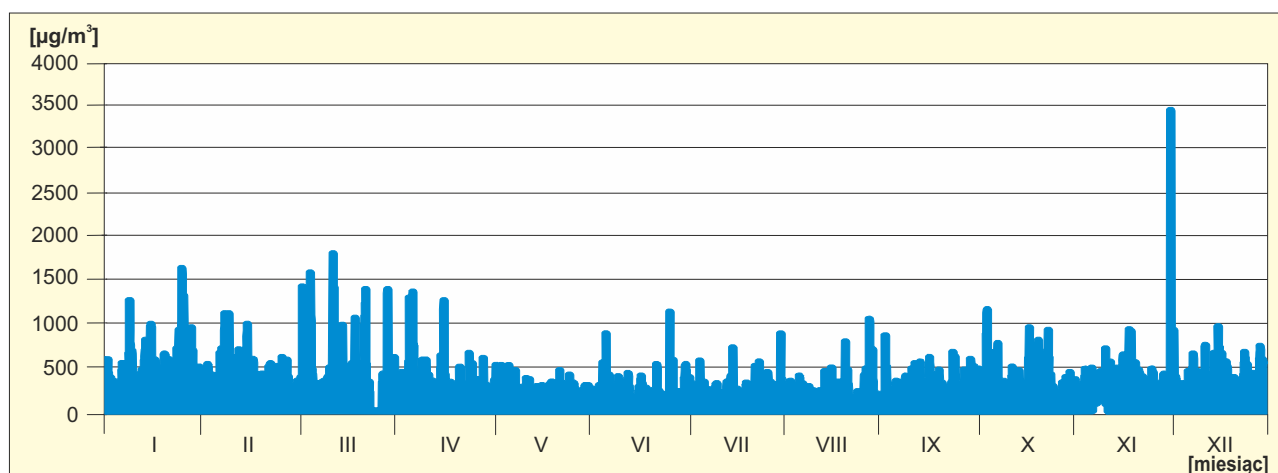
Rys. 3.10. Przebieg stężeń jednogodzinnych CO na stacji w Poznaniu, ul. Polanka w 2013 roku
