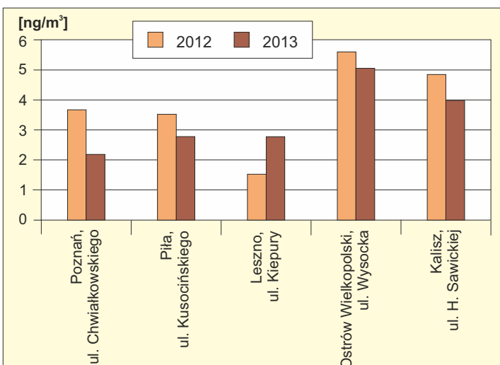
Rys. 3.13. Stężenia średnie dla roku benzo(a)pirenu w roku 2012 i 2013 na wybranych stanowiskach w województwie wielkopolskim /wg WIOŚ w Poznaniu/
