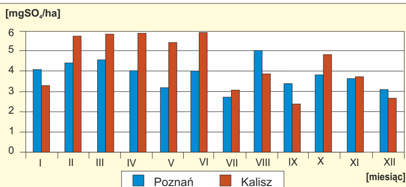
Rys. 3.2. Miesięczne zmiany zawartości siarczanów w opadach atmosferycznych w 2013 roku w Poznaniu i Kaliszu /wg IMGW/
