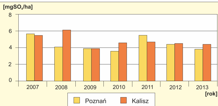
Rys. 3.3. Zmiany zawartości siarczanów w opadach atmosferycznych w latach 2007-2013 w Poznaniu i Kaliszu /wg IMGW/
