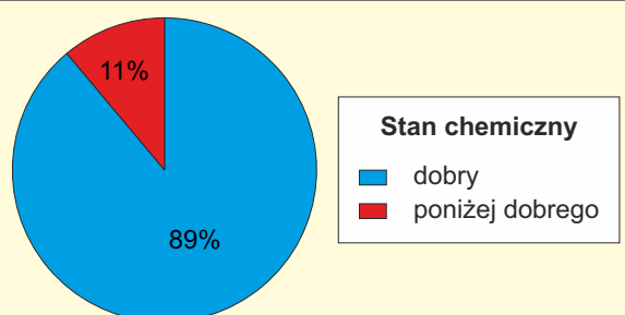
Rys. 4.9. Ocena stanu chemicznego JCW jeziornych w 2013 roku /wg WIOŚ/
